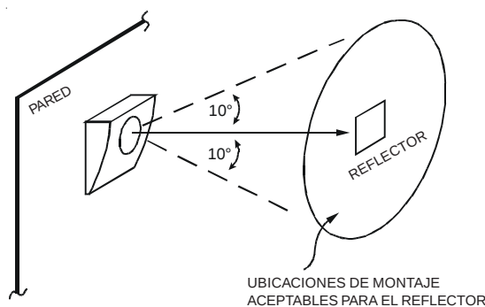
El reflector se monta directamente en la pared utilizando los cuatro orificios de montaje, uno en cada esquina. Se debe instalar de manera que la plancha del reflector quede perpendicular al campo visual óptico de la unidad con transmisor/receptor. La tolerancia máxima para las posiciones de montaje que no son perpendiculares es de 10°. Si no es posible obtener esta tolerancia, es necesario utilizar la base MMK, consulte las instrucciones de MMK si desea más detalles.
